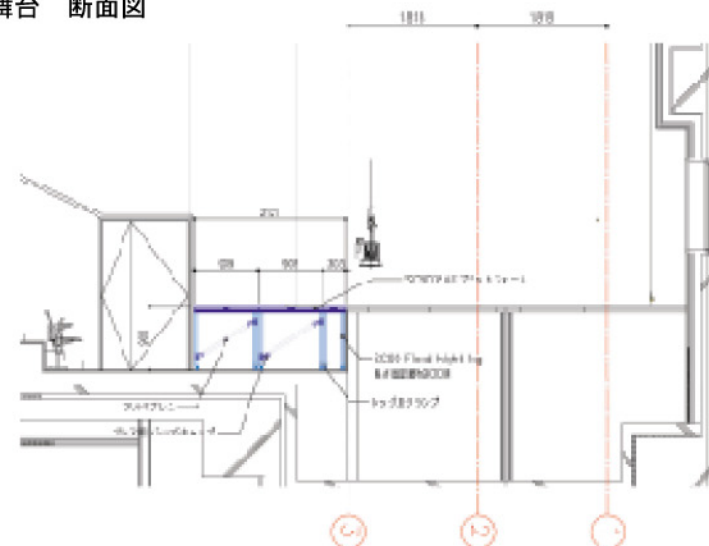
基本舞台 断面図
